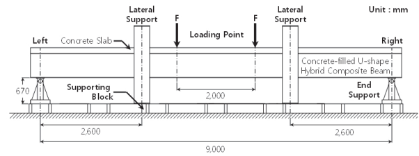
Fig. 8. Test setup
